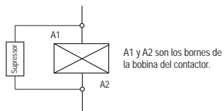
Esquema de conexión de supresores en contactores
